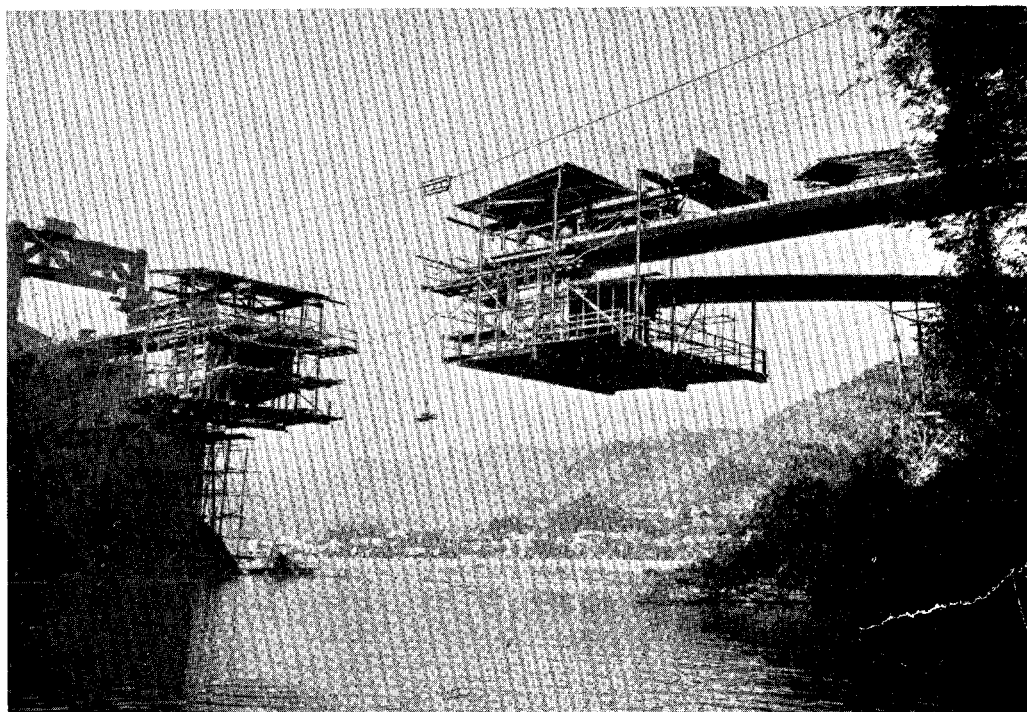
接合間近かき片持橋桁
