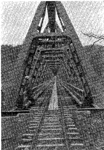
森林軌道三弦橋 (ダム サイト上流)
