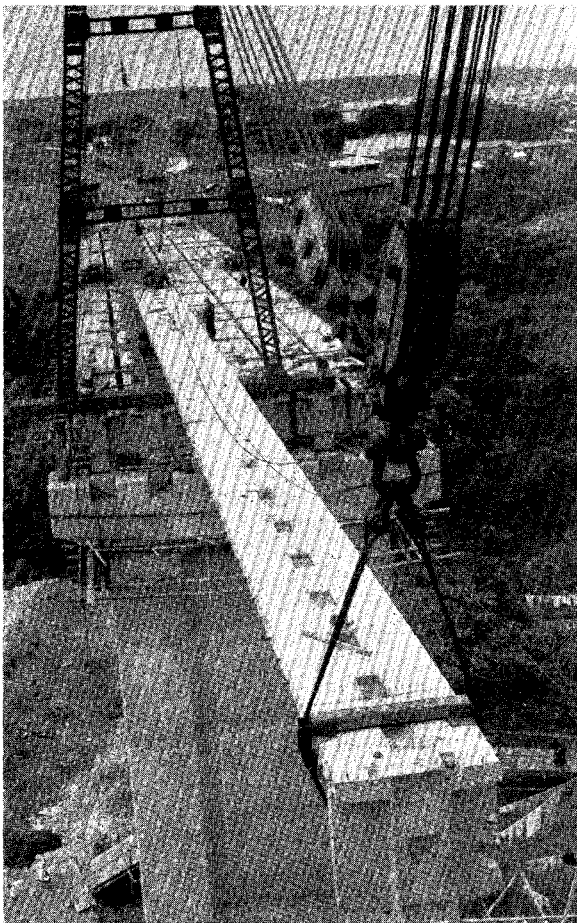
陸橋架設中の PC 桁俯瞰観
