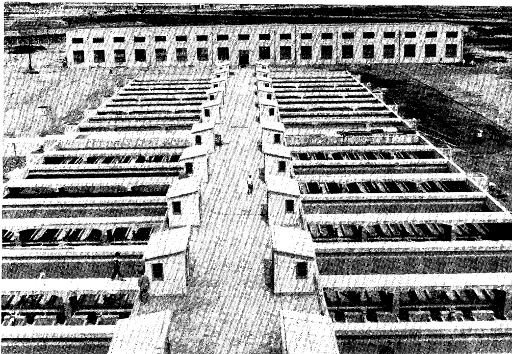
急速濾過場の回転式表面洗滌装置
