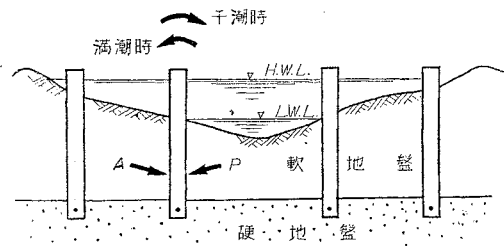
図-2 断面略図
