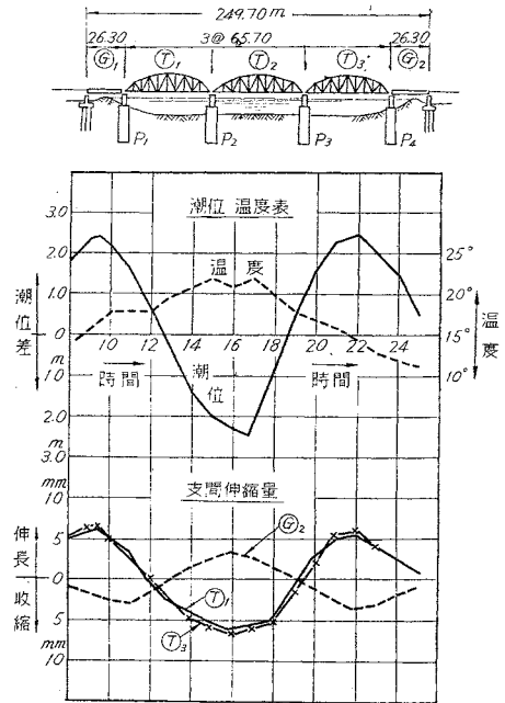
図-3 径間伸縮測定図 (住之江橋)
