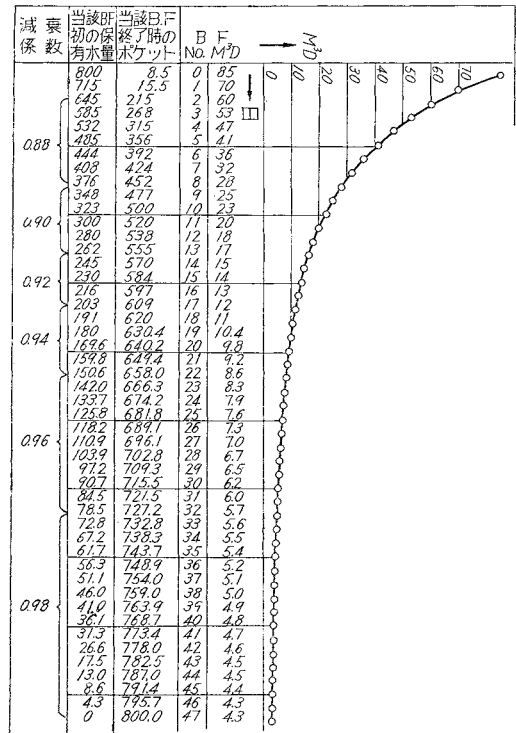
図-1 基底流曲線(岡山県旭川第一ダム)
