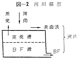
図-2 河川模型
