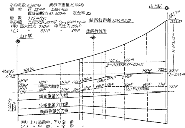
図一2 運転示力図
