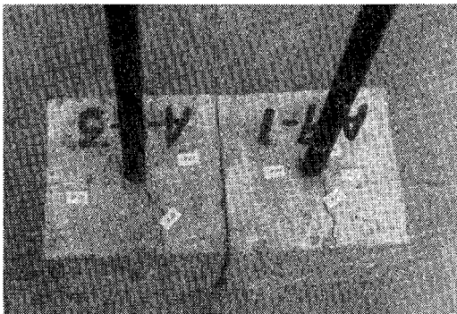
写真-2 コンクリートのキレツ発生状況 (直流20V陽極的荷電、塩カル1%)
