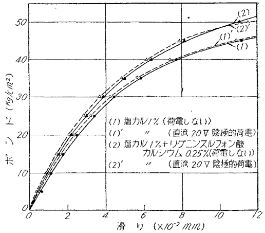
図-14 直流陰極的荷電のボンドと滑り (塩化カルシウム系コンクリート)
