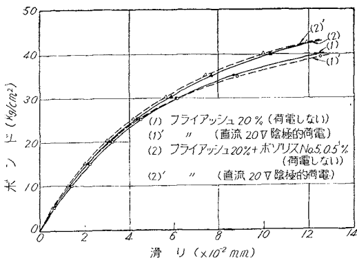
図-18 直流陰極的荷電のボンドと滑り (フライアッシュ系コンクリート)
