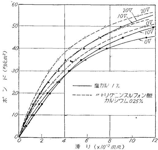
図-13 直流陽極的荷電のボンドと滑り (塩化カルシウム系コンクリート)
