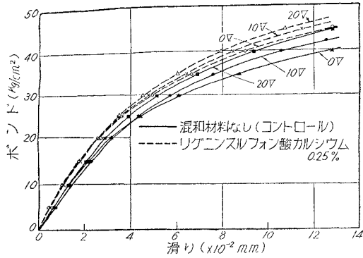
図-11 直流陽極的荷電のボンドと滑り
