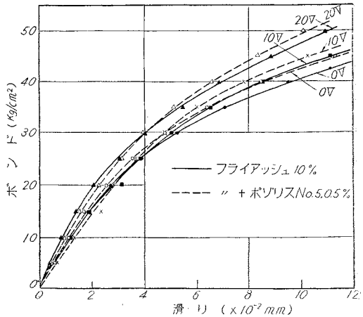
図-15 直流陽極的荷電のボンドと滑り (フライアッシュ系コンクリート)
