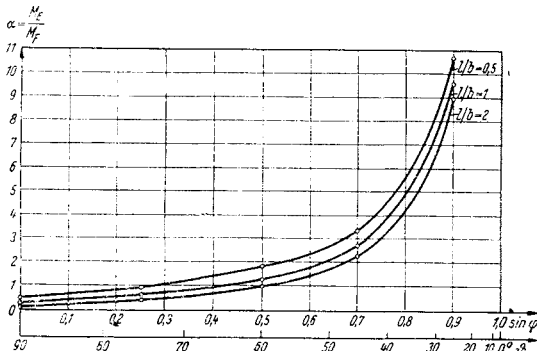
図-4 荷重状態Aによる \alpha の値
