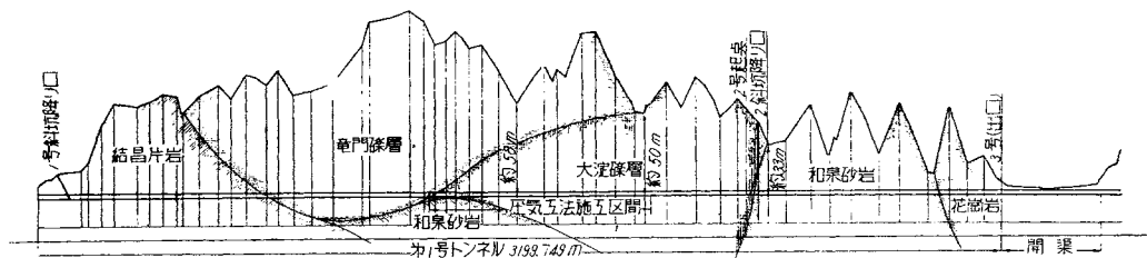
図-1 縦断面図
