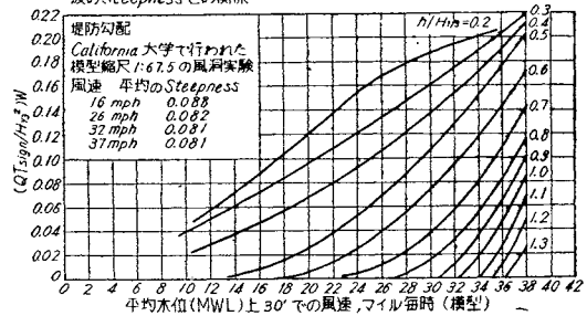
(b) 堤防高さも色々変えた場合の風的作用により加わる越水量
