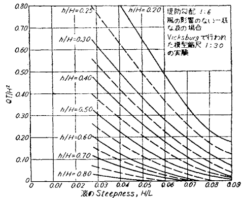
(a) 平均水位(MWL)上の堤防高さも色々変えた場合の波による越水量と波の Steepness との関係
