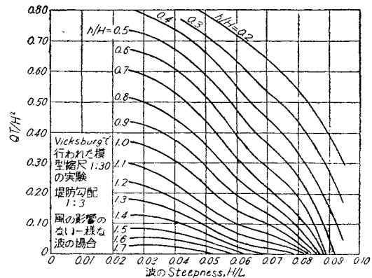
(a) 平均水位(MWL)上の堤防高さも色々変えた場合の波による越水量と波の Steepness との関係
