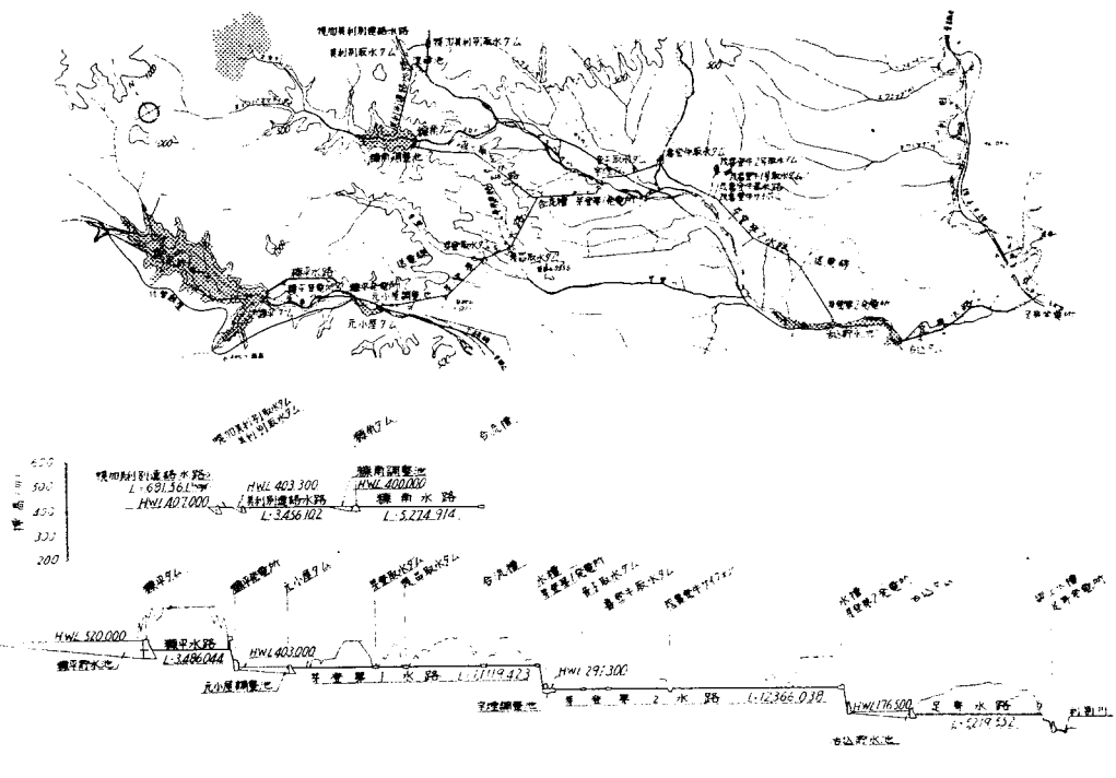
図-1 糠平系計画平面図および縦断面図
