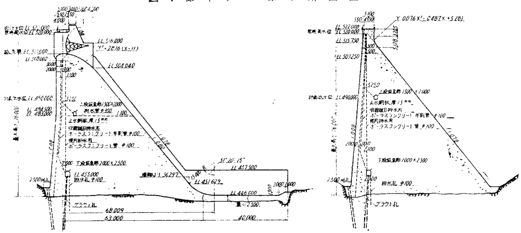
図-4 糠平ダム標準断面図
