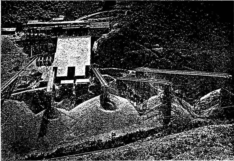
篩分工場並骨材貯蔵所 (朝鮮軍司令部許可済)
