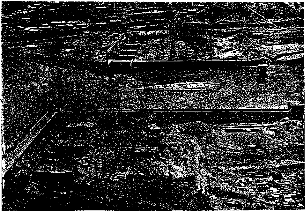
兩岸締切壁内掘鑿及コンクリート打込作業 (朝鮮軍司令部許可済)
