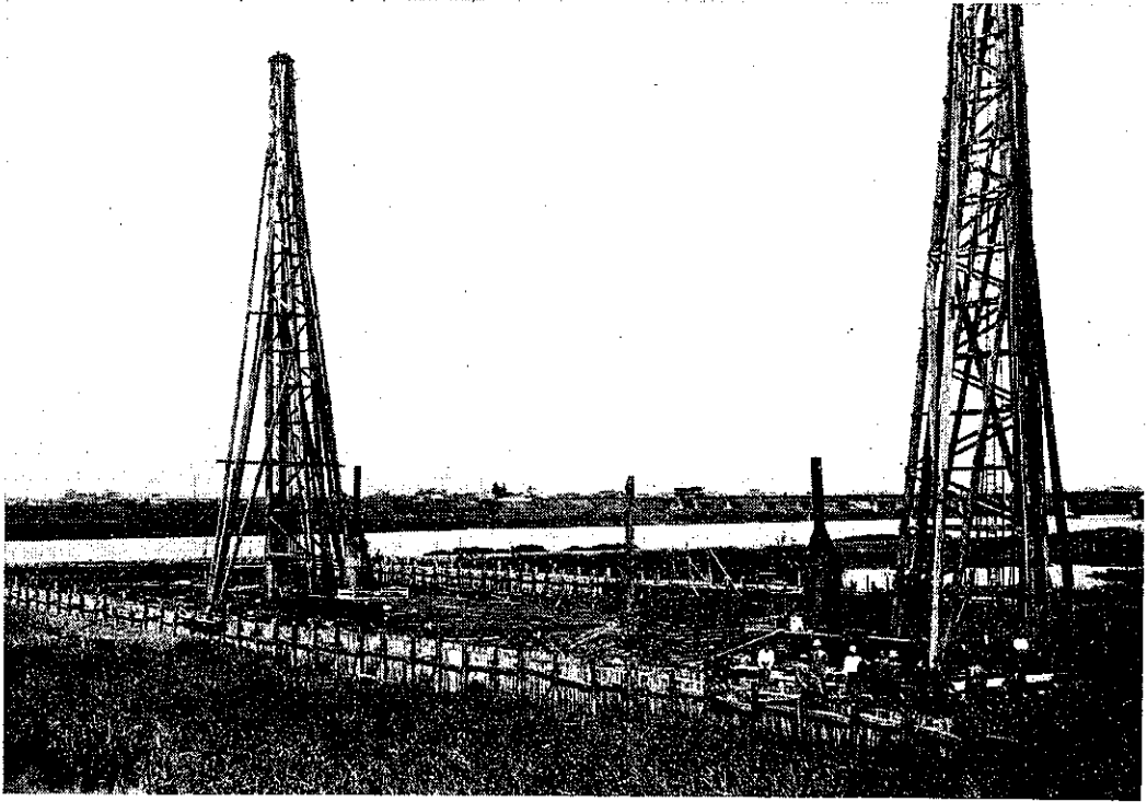
東京府四ツ木橋基礎杭(ペDESTAL混凝土杭 杭徑 50.8 糎杭長 20 米, 合成松杭 杭徑 24 糎杭長 9 米)工事現場作業實況
