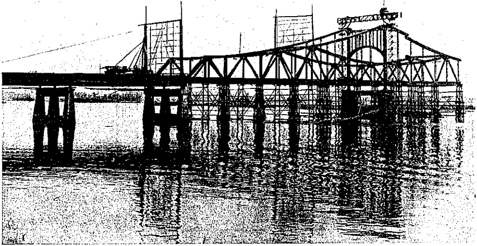
トラスの架設を東京側より望む
