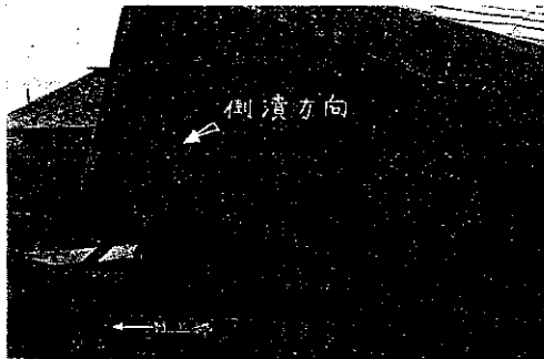
図-3. 渡島當別驛別貨物上家の倒壊 (其の 1)
