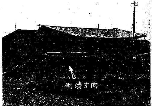
図-4. 渡島當別驛別貨物上家の倒壊 (其の 2)
