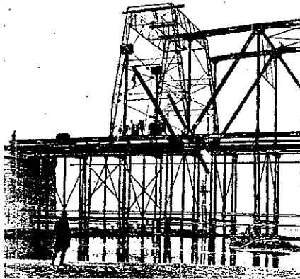
構桁架設中
