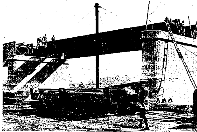
鋼 鈹 桁 架 設 中
