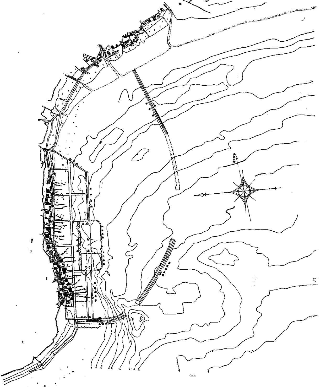
瀨漁港平面圖
