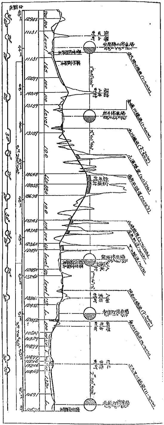
房總線勝山北條間工事中心線路一覽圖
