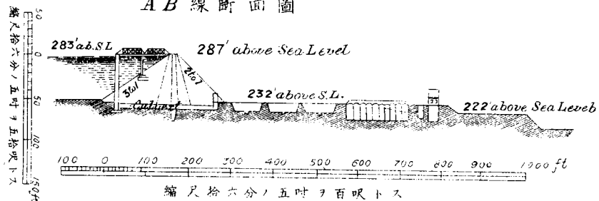
AB線断面圖
