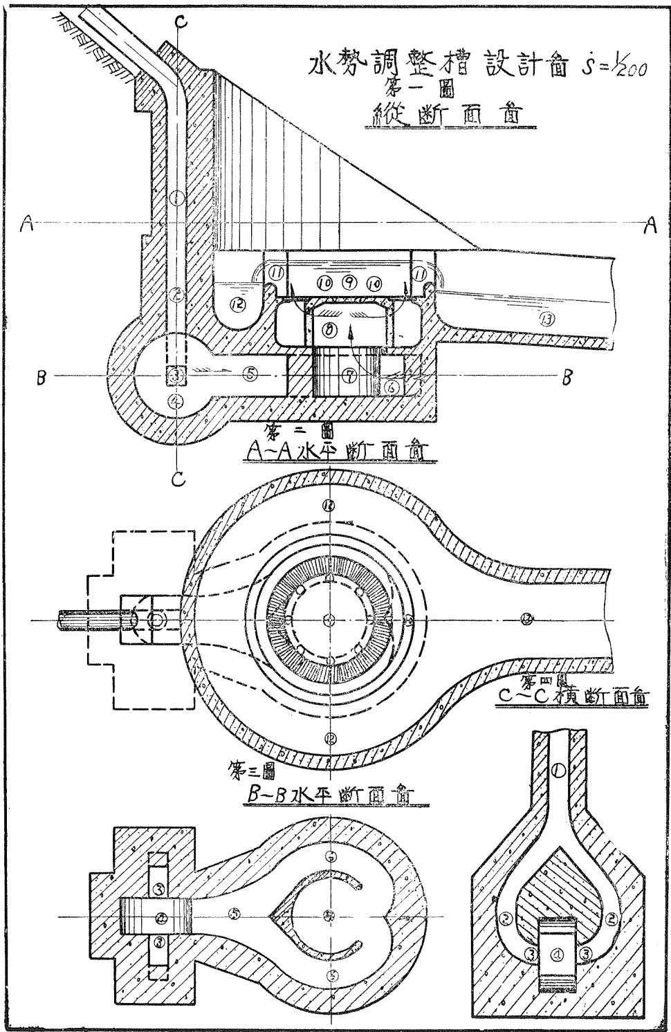
圖 1.2.3.4. 水勢調整槽設計圖。
