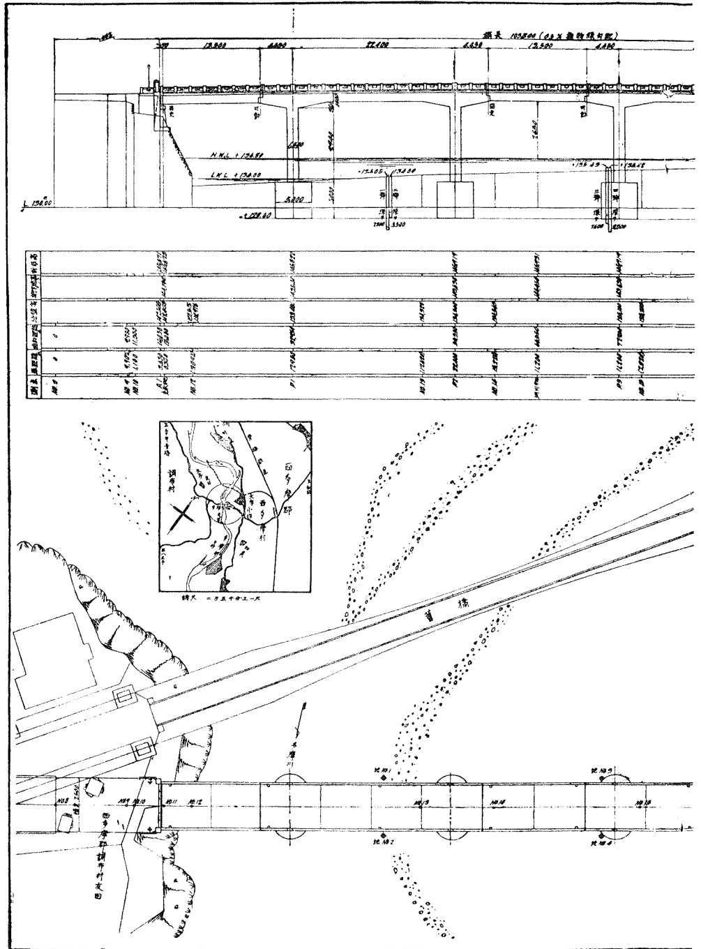
圖 1. 東京府多摩川橋平面及側面圖。
