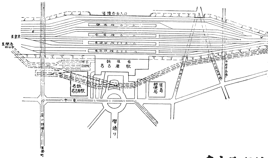
圖1. 線路平面圖
