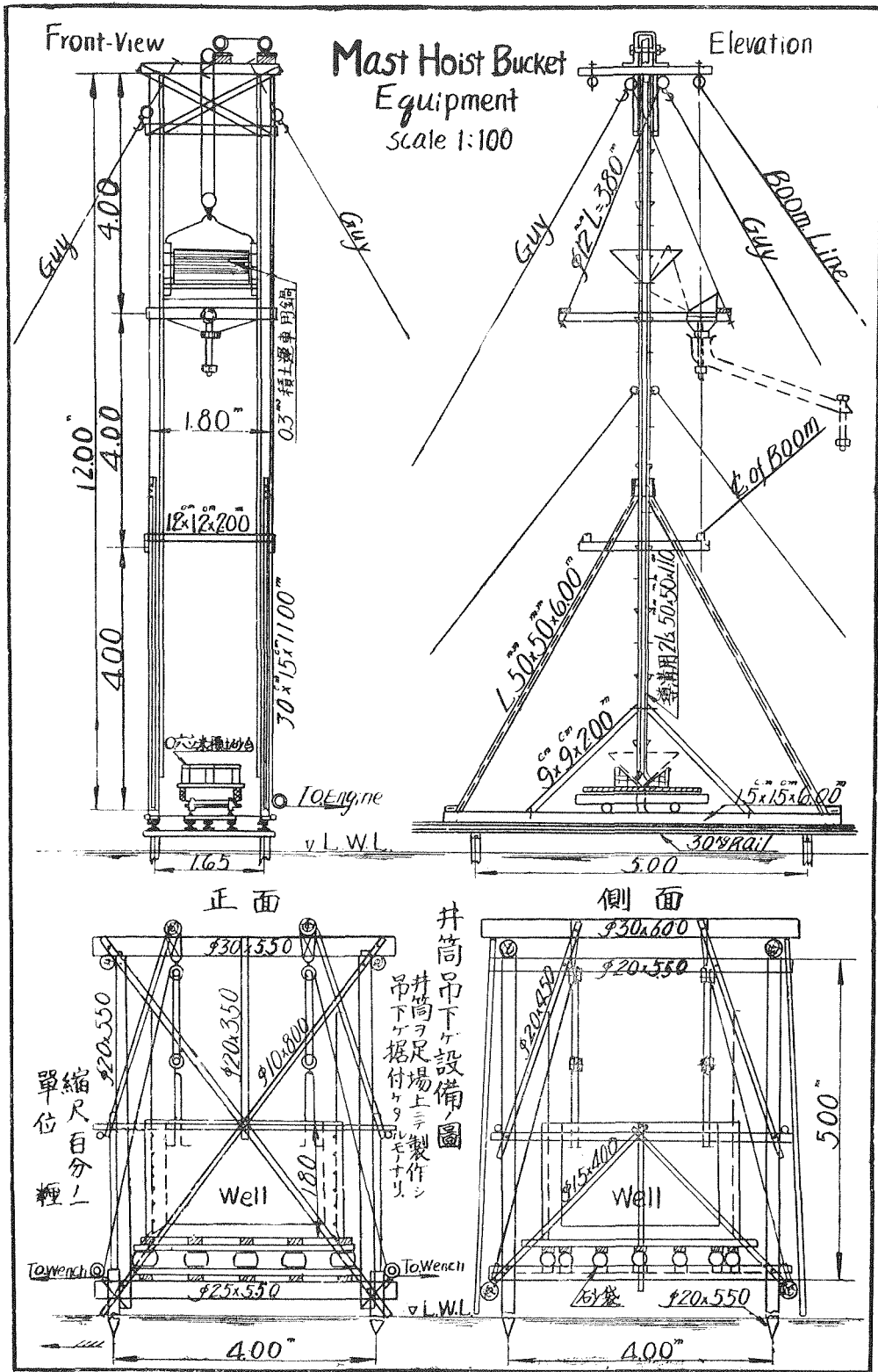
14. コンクリート送達及井筒吊下設備圖。
