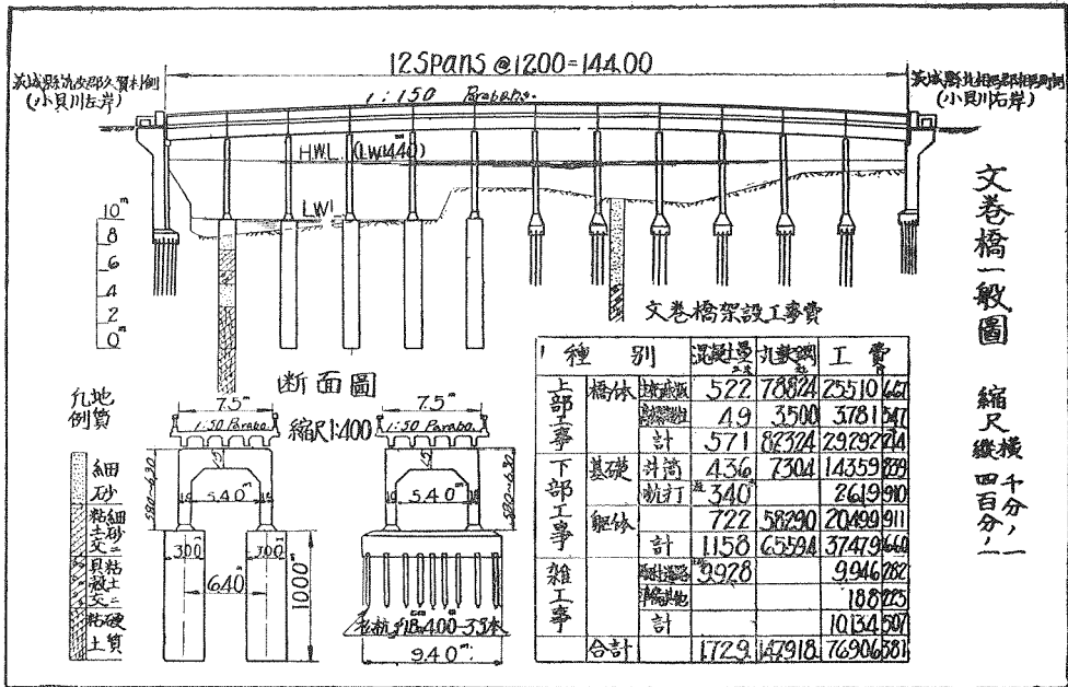
1. 文巻橋一般圖
