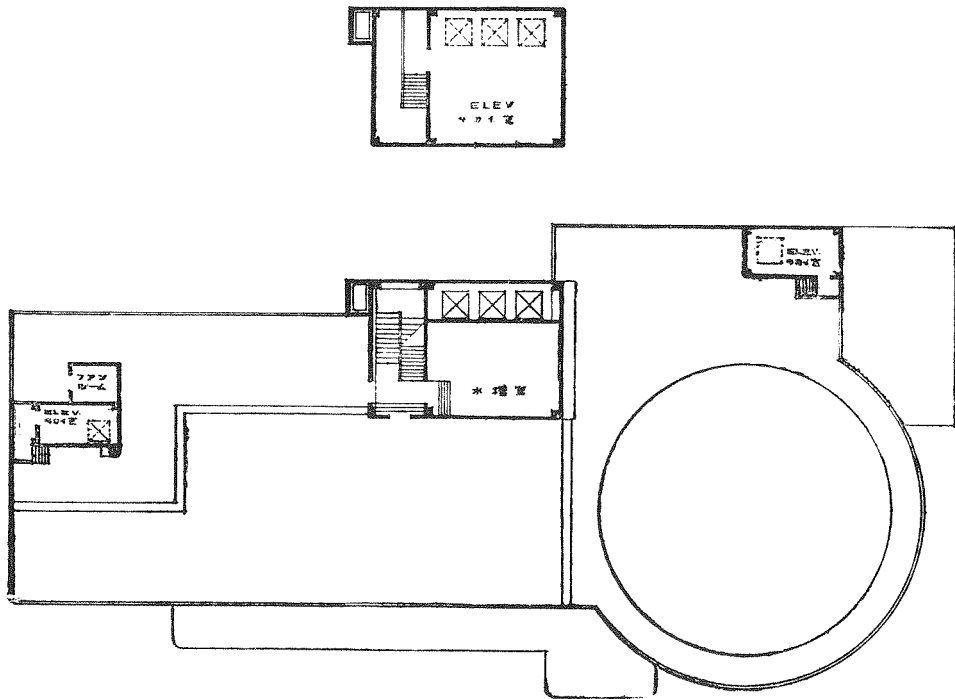
12. 東日會館屋階平面圖。
