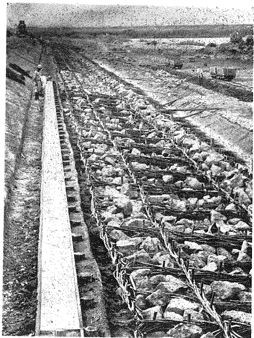
31. 護岸根固め沈床（粗朶）施工状況。
