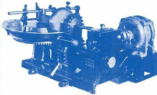
商工省標準「セメント混合機」 (スタインブリツクシエメルツアー型)
