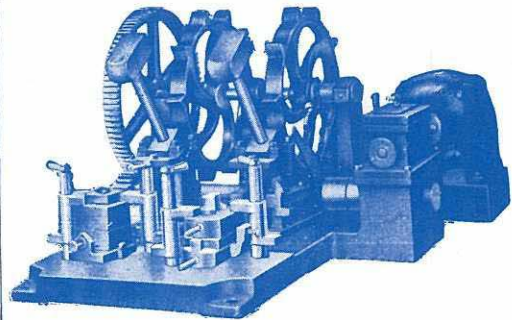
商工省標準鐵繩機(ペーメマルテンス型)
