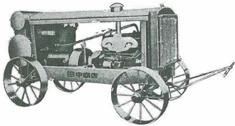
瓦斯倫機關直結 可搬式空氣壓縮機
