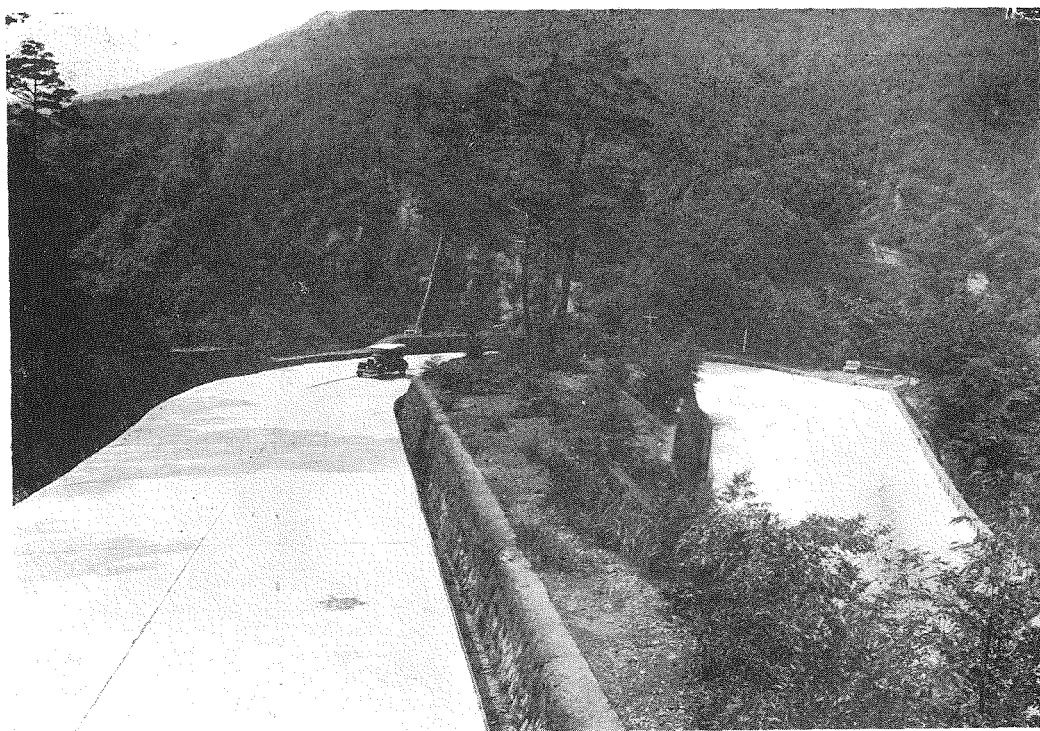
(1) 竣工せる 91 號國道・神奈川縣足柄下郡溫泉村大字大平臺。
