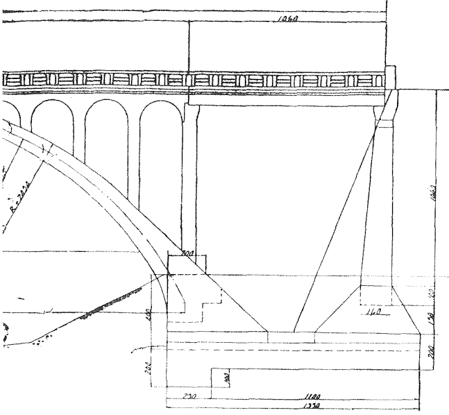
右岸断面图
