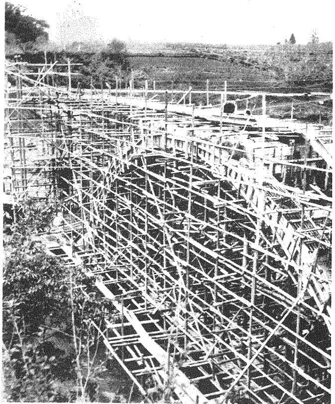
(3) 兩橋拱徑間架設足場正面。
