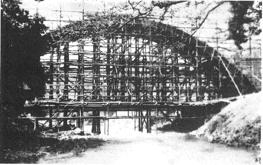
(2) 兩橋拱徑間架設足場側面。
