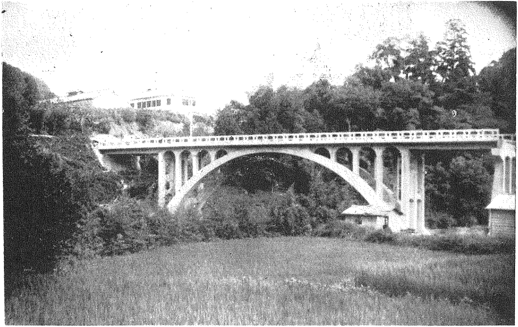
(1) 竣工せる兩橋全景。
