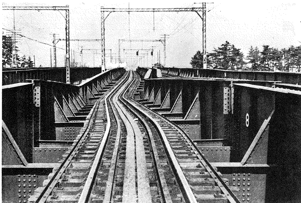
武庫川橋梁(立花甲子園口間)の被害
