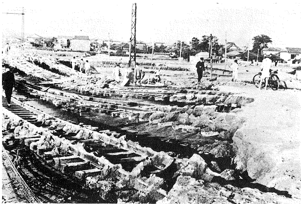
攝津本山住吉間線路の被害状況
