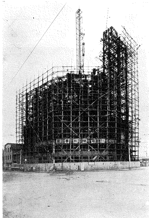
(2) 清水組で施工中の大阪市 電気局電気科学館。
