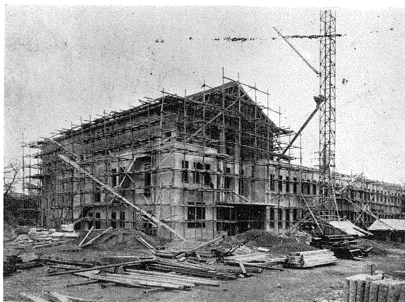
(1) 大阪青年塾で松村組 の手により工事中。
