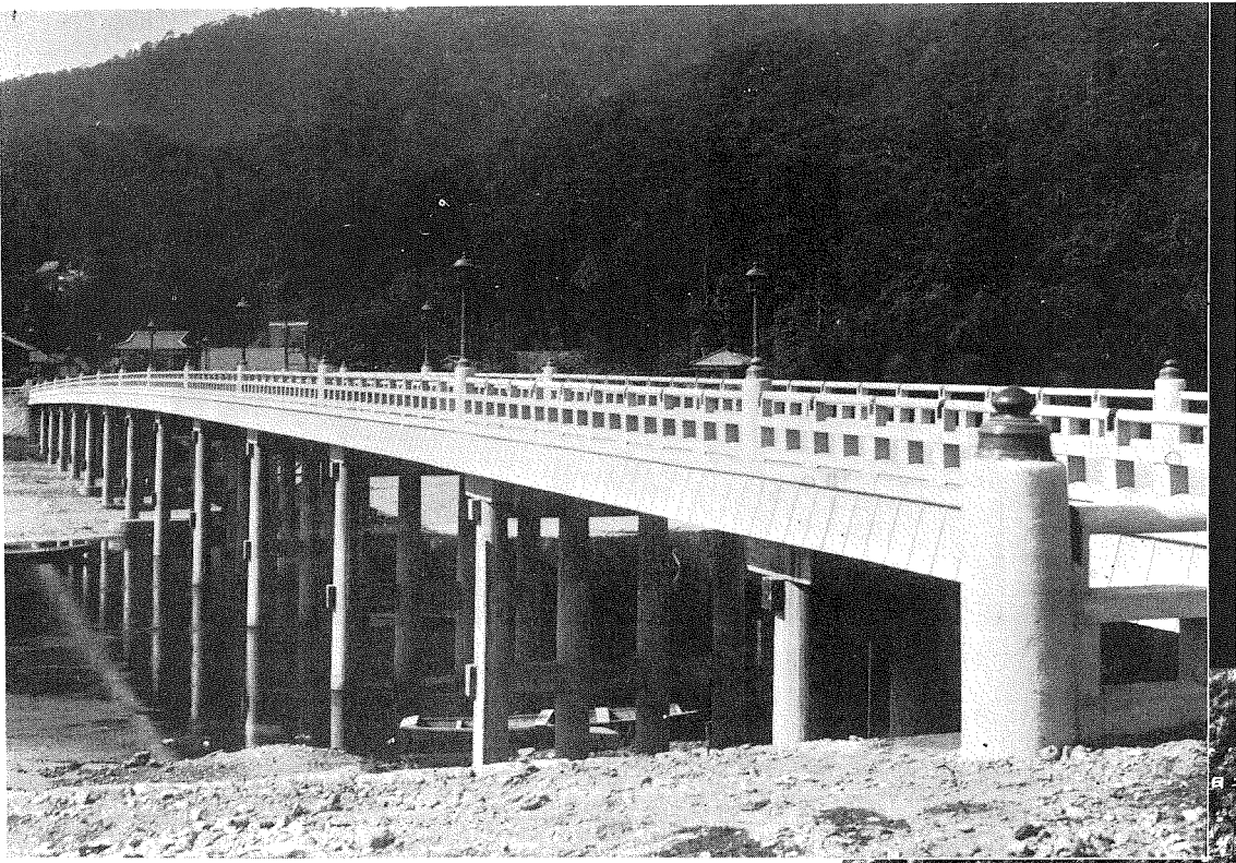
(1) 山口縣岩國町の臥龍橋全景。
