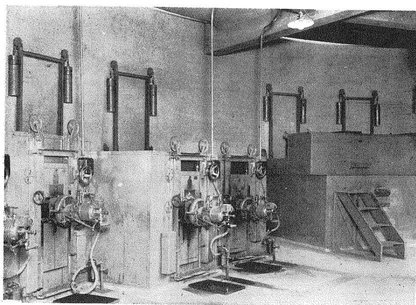
(5) 八事火葬場 作業室内部。
