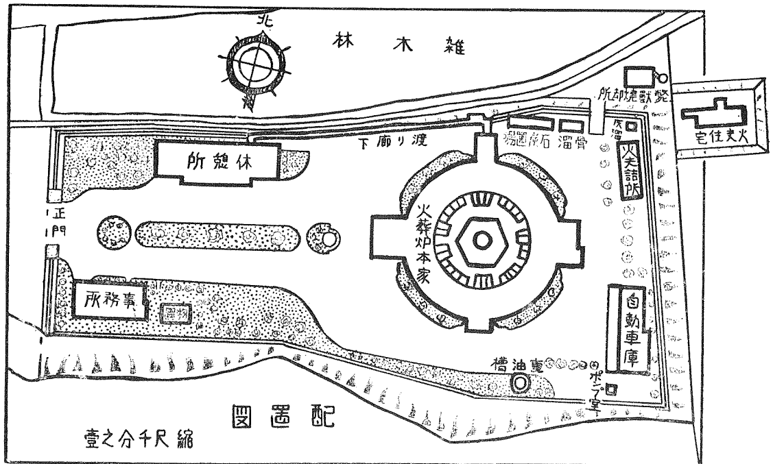
(3) 八事火葬場配置圖。
