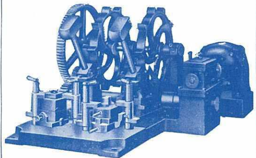
商工省標準鐵礮機(ベーメメルツァン型)
