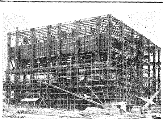
關西共同火力發電株式會社 尼崎發電所鐵骨
