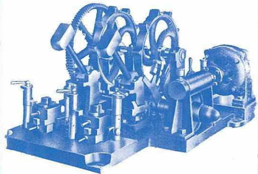
商工省標準槌機(ペーメルテンス型)
