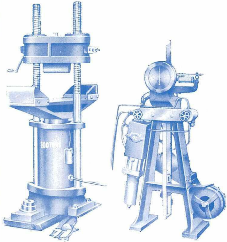
東京衡機アムスラー型壹百磅耐壓及彎曲試驗機
