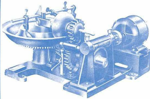
商工省標準「セメント混合機」 (スタインブリツクシユメルツアー型)
