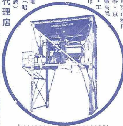
セメント衡量機並にバイブレーションを常備せる改良E型機
