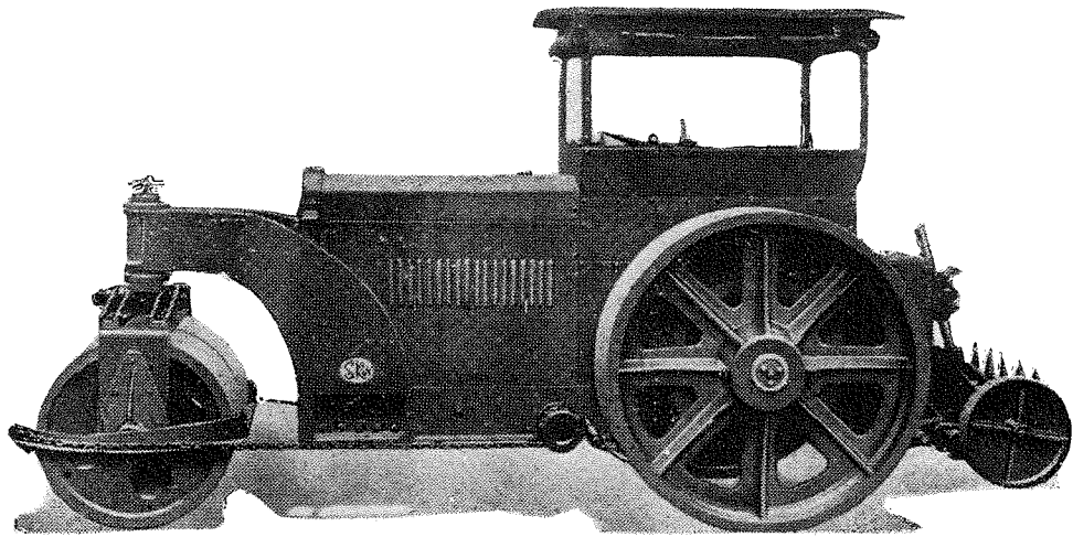
青森市役所納入 十噸ロードローラー
