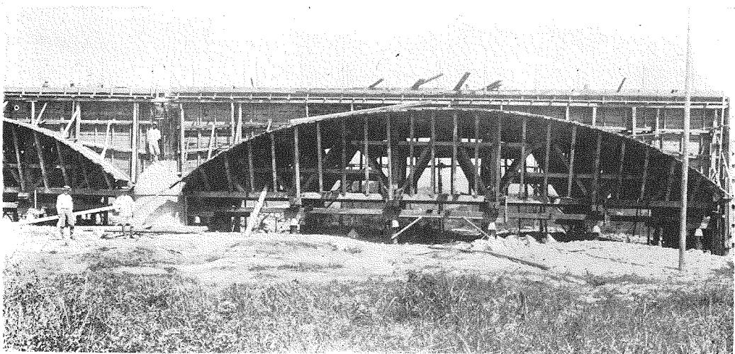
(2) 正條橋アー チのセンターリ ング。
