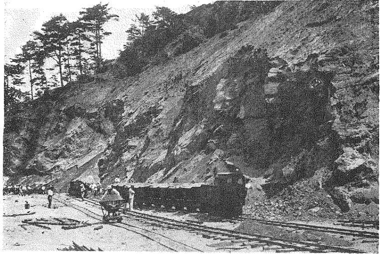
4 廣島縣佐伯郡觀音 村地内觀音及五日 市路床工事土取場 (岩戸山切取作業 中の景) (6.7.7)
