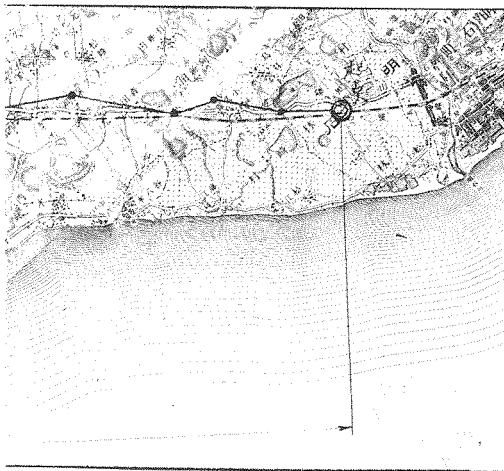
(右上) 岡山縣國道第2號線工事個所平面圖。 (左) 和歌山縣國道第15號線工事個所平面圖。 (中) 和歌山縣國道第16號線工事個所平面圖。 (下) 廣島縣國道第2號線工事個所平面圖。
