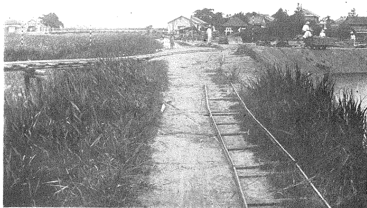
2 同上、白石橋架設 位置現況、嵯々瀬 川右岸上流より舊 白石橋を望む。 (6.6.28)
