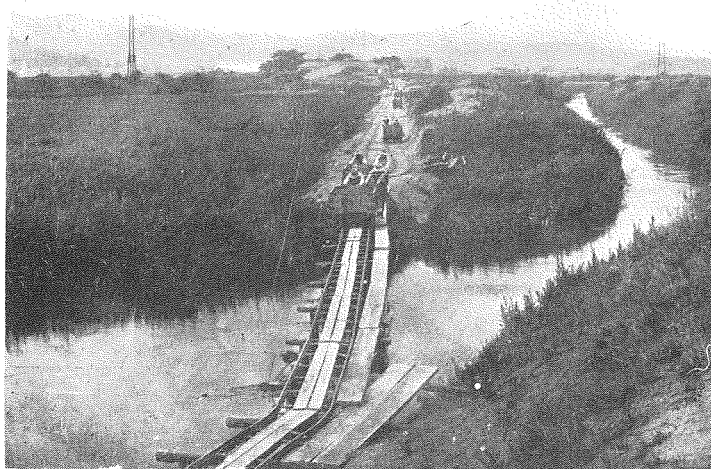
1 岡山縣國道第2號 線工事土運搬の實 況。(6.6.28)
