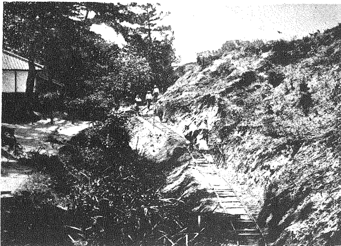
5 兵庫縣國道第2號 線工事、延軌道條 布設中の實況(明 石郡大久保村大字 松蔭) (6.6)
