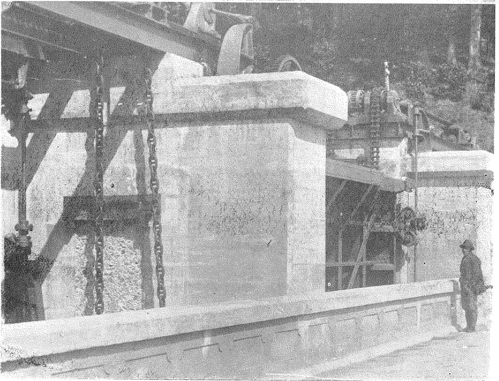
(28) 門扉上下装置(上流より)
