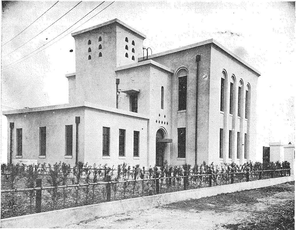
第9圖 江尻電話中繼所全景
