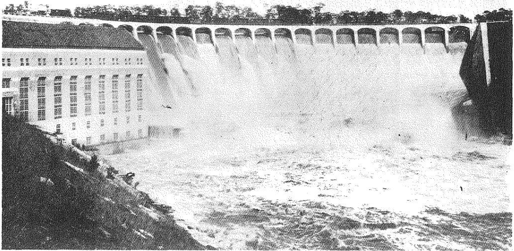
第1圖 マルチンダムの補助堰堤が本堰堤より溢流する水勢を減殺しつつある景
