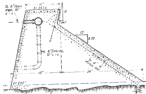
第2圖 補助堰堤の横断面圖、本堰堤より流下する水は傾斜の緩なる面に當る。
