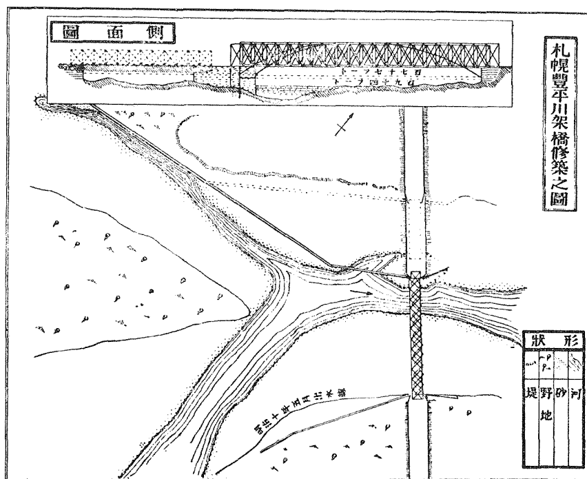
(2) 明治十年來人土木技師ホイラー氏の設計圖
