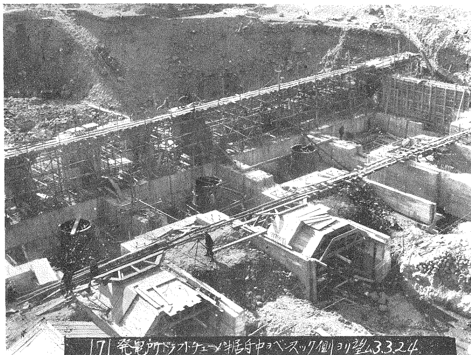
(1) 已に施工せる基礎上に鐵筋及型板組立中を示す
