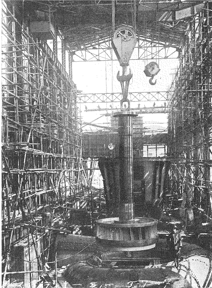
(3) 水車取付中 ランナーをスパイラルケーシングへはめ込むところ。
