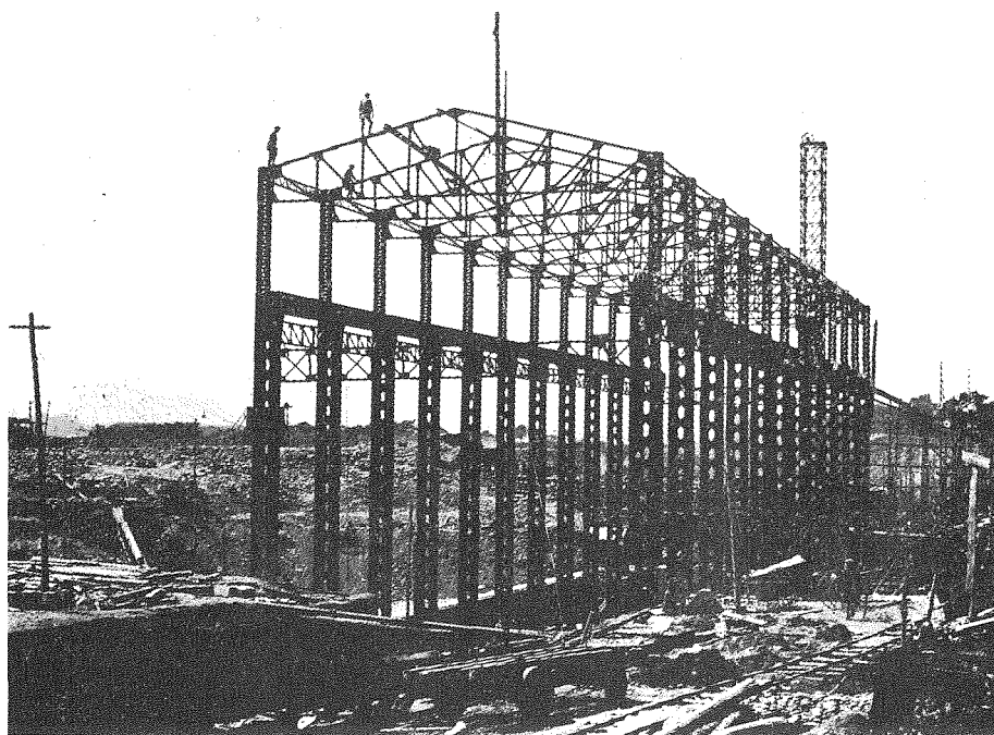
(2) 發電所鐵骨組立完成
