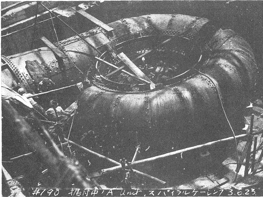
(5) 水車据付中
