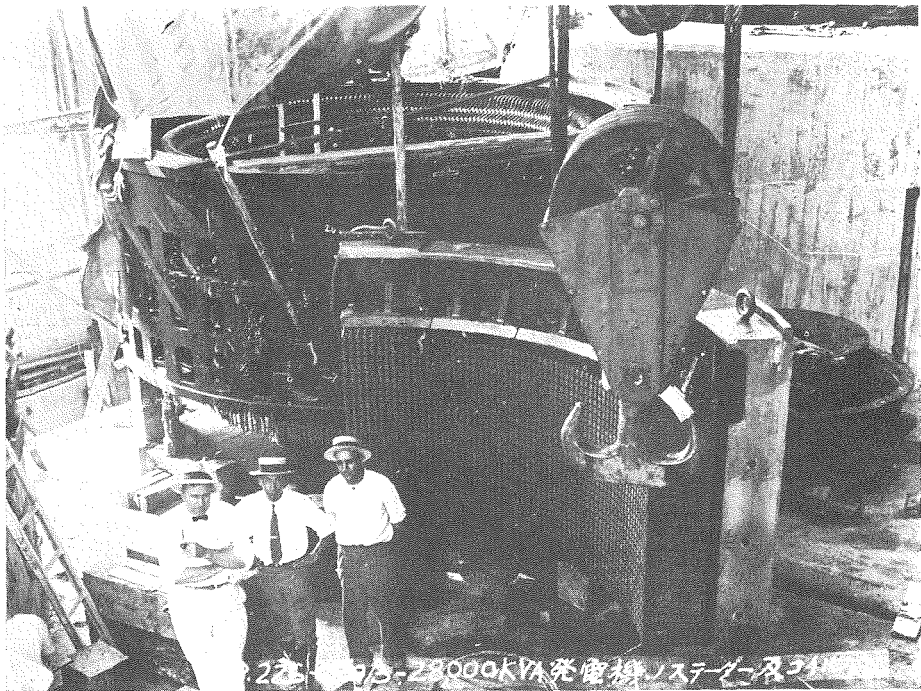
(6) 發電機据付中
