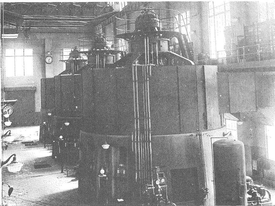
(8) 据付完成せる3臺の28,000 K.V.A.發電機
