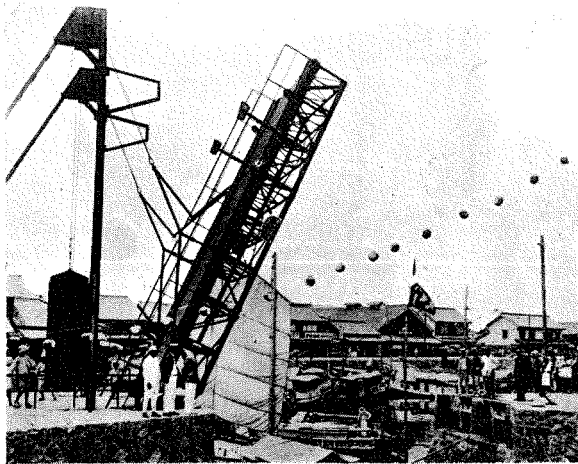
坂出町の跳開橋(本年七月竣工)
