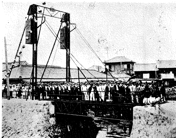
香川縣坂出町に本年七月竣工したる跳開橋 (設計、山本卯太郎)
