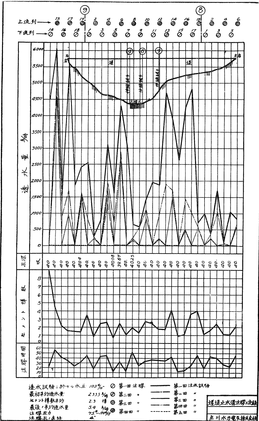
(9圖) 小牧堰堤止水溝注膠工記錄
