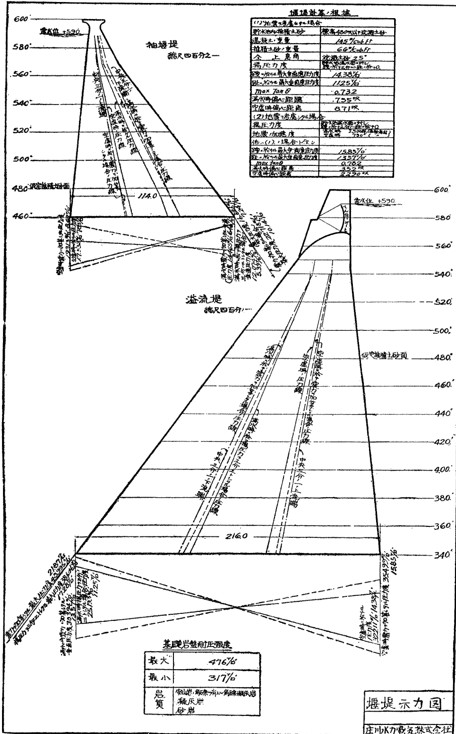
(6圖) 小牧堰堤示力圖
