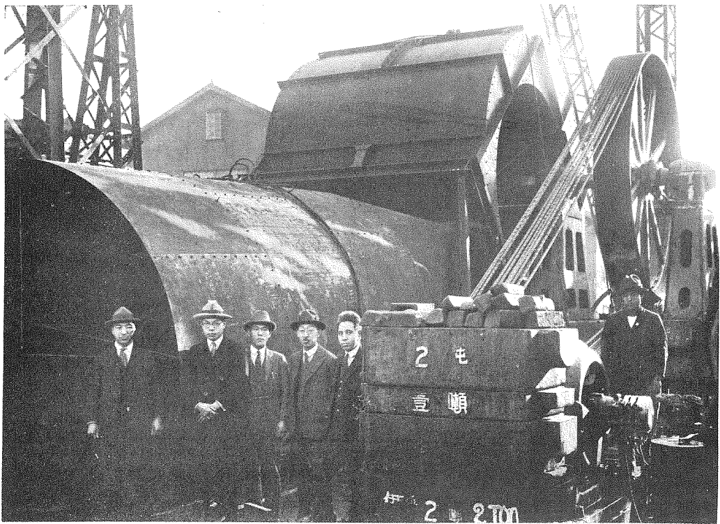
東山トンネルの排煙装置ファン（昭和三年四月落成）
